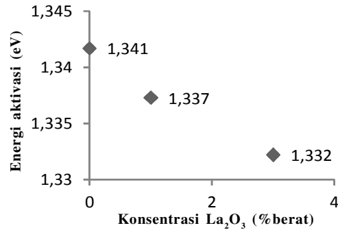
Gambar 7. Grafik energi aktivasi elektrolit padat CSZ terhadap konsentrasi La 2 O 3
