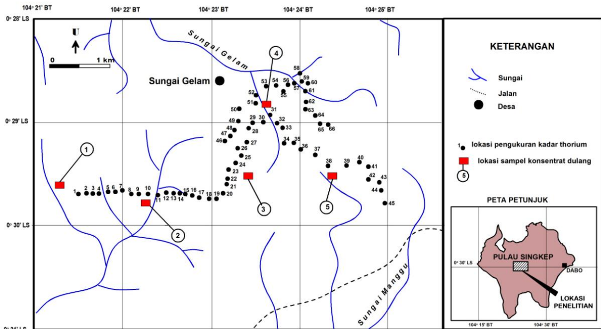
Gambar 2. Peta lintasan pengukuran kadar torium dan lokasi sampel konsentrat dunglai di kawasan laterit bauksit.
