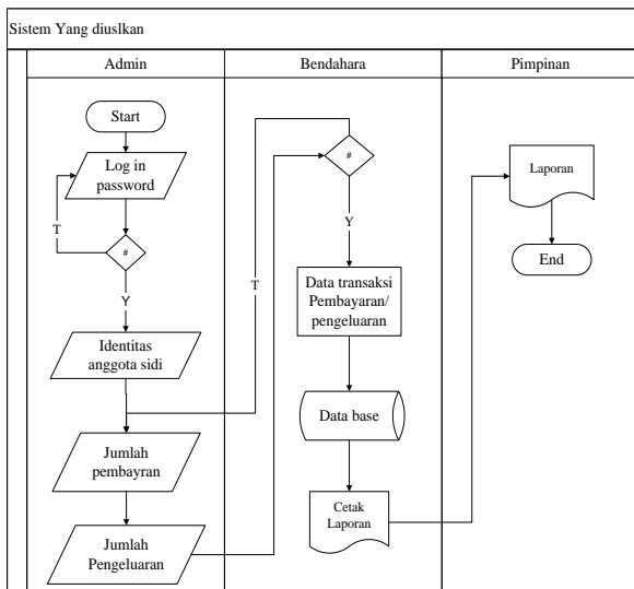
Gambar 3. Flowchart Sistem Yang Diusulkan
