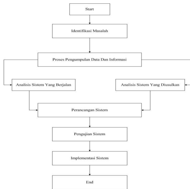
Gambar 1. Kerangka Penelitian
