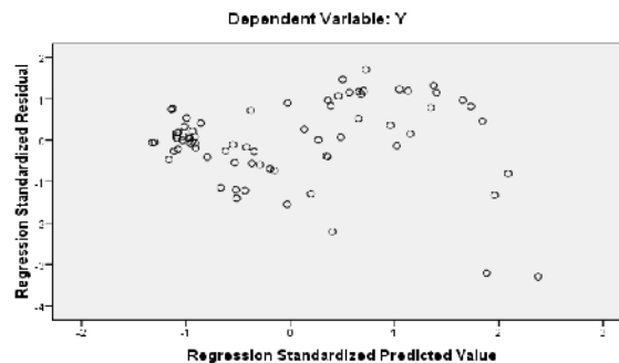
Gambar 5.1 Uji Heteroskedastisitas
