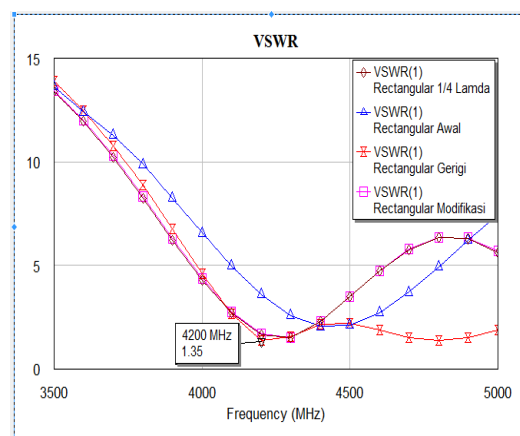
Gambar 7. Grafik VSWR antenna mikrostrip rectangular gerigi dengan 13 slit
