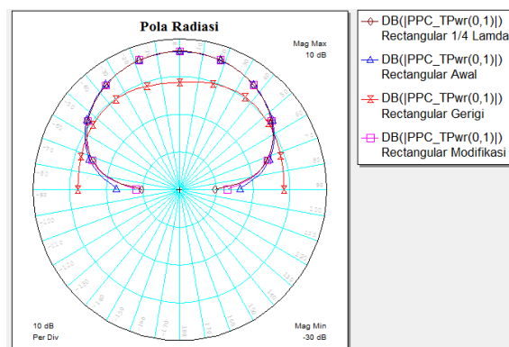
Gambar 9. Grafik pola radiasi antenna mikrostrip rectangular gerigi dengan 13 slit
