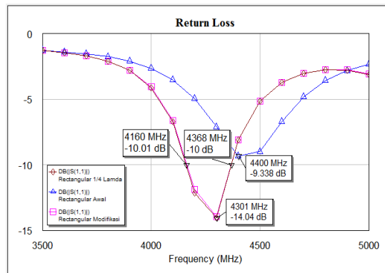
Gambar 5. Grafik return loss untuk ketiga jenis antenna mikrostrip rectangular
