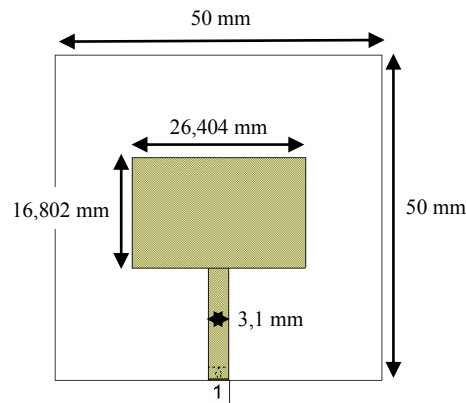
Gambar 2. Antena mikrostrip rectangular modifikasi
