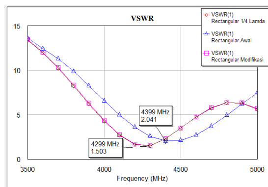
Gambar 4. Grafik VSWR untuk ketiga jenis antena mikrostrip rectangular
