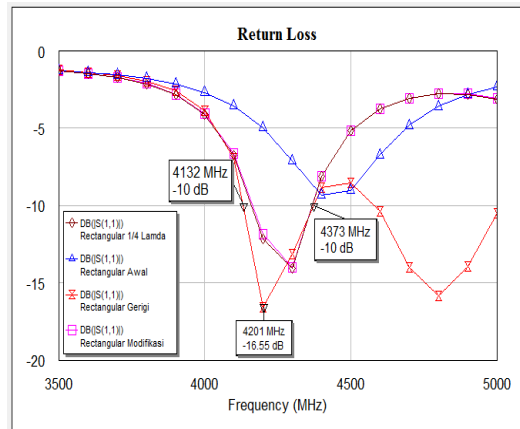
Gambar 8. Grafik return loss antenna mikrostrip rectangular gerigi dengan 13 slit
