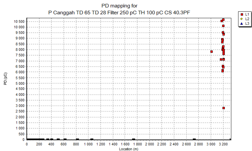
Gambar 8. Penyulang Cangah Gardu TD 65 ke Arah TD 28
