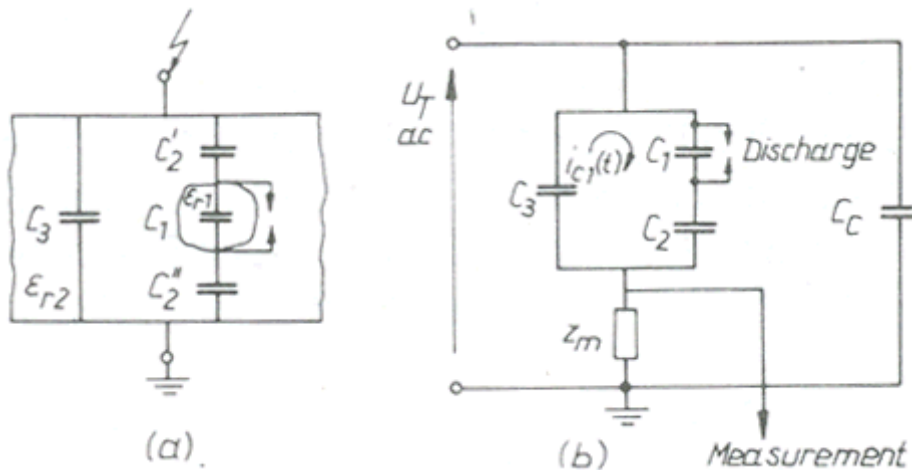
Gambar 1. Rangkaian Ekivalen Rongga Pada Kabel
