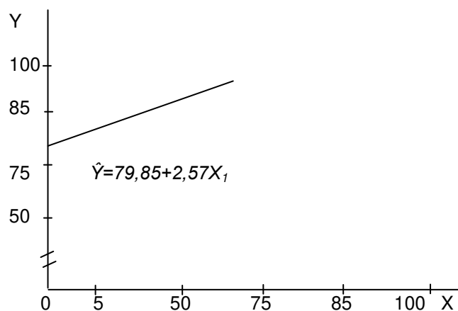
Gambar 1. Garis Regresi Hubungan Antara Implementasi Manajemen Berbasis Sekolah (X) dengan Efektivitas sekolah (Y)
