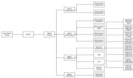
Gambar 3.11 Perancangan Struktur
