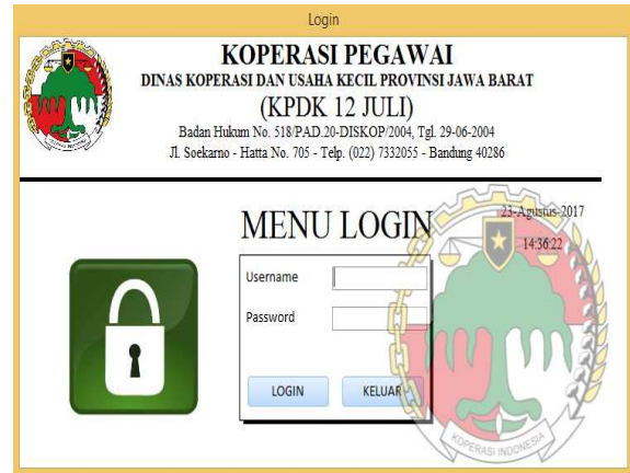
Gambar 4.2 Halaman Login
