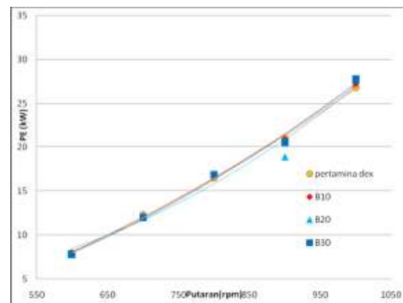
Gambar 3 Grafik daya vs rpm pada balast load
