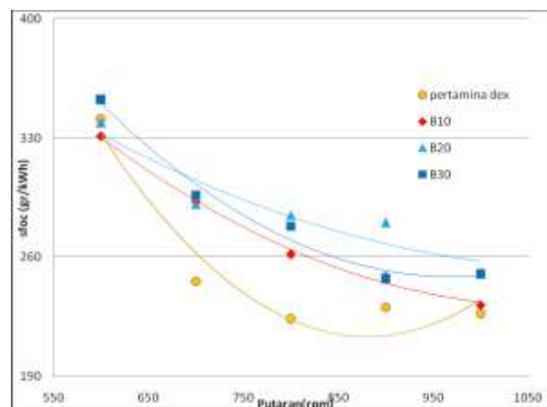
Gambar 5 Grafik sfoc sebagai fungsi rpm pada balast load
