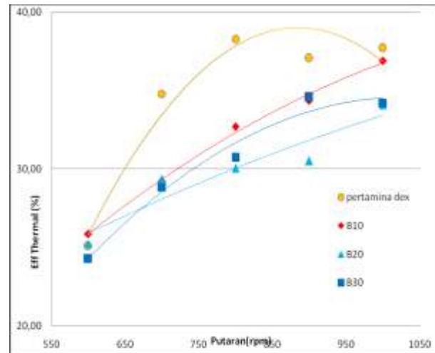
Gambar 6 Grafik eff thermal sebagai fungsi rpm pada balast load
