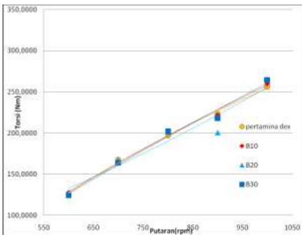
Gambar 4 Grafik torsi sebagai fungsi rpm pada balast load
