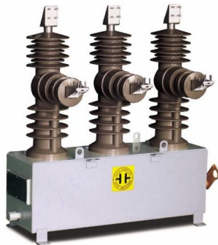
Gambar 2.2 Recloser Entec EVRC 2A
