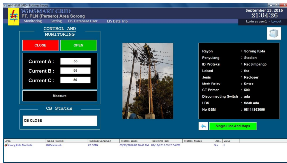
Gambar 4.3 Detil Recloser Simpang 5
