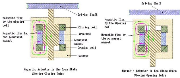
Gambar 2.4 Prinsip magnetik pada operasional penggerak
