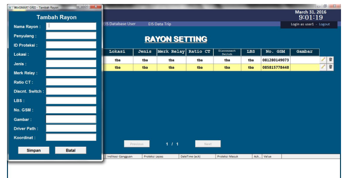
Gambar 3.9 Tambah Rayon
