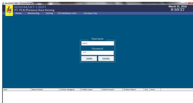
Gambar 3.2 Login
