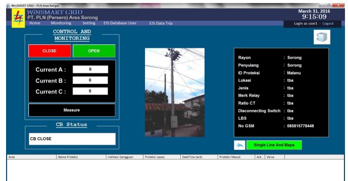
Gambar 3.4 View Detil
