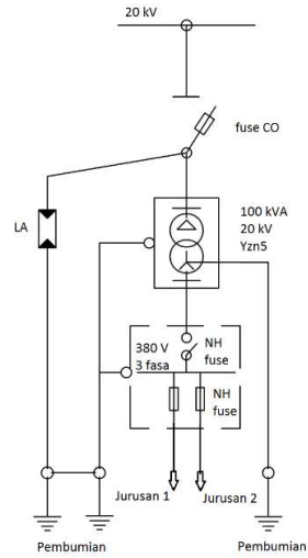
Gambar 3.2 Single Line Trafo Distribusi 100 kVA Dua Jurusan
