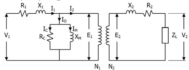
Gambar 2.3 Rangkaian Ekuivalen 1
