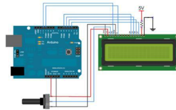
Gambar 4.12 Rangkaian LCD
