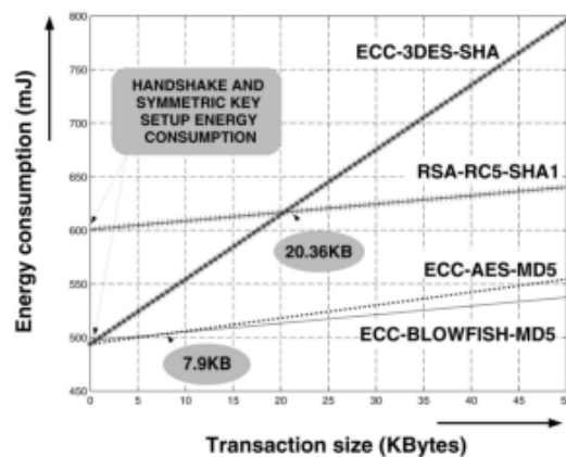
Gambar 2. Konsumsi energi selama SSL Handshake
