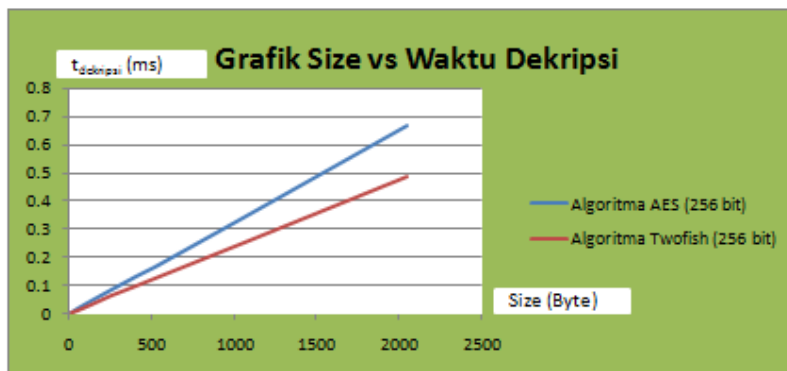
Gambar 13 Grafik size vs waktu dekripsi
