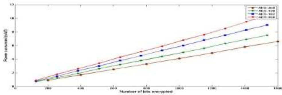
Gambar 5. Konsumsi daya vs jumlah bit yang dienkripsi AES untuk panjang kunci yang bervariasi
