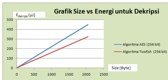
Gambar 17. Grafik konsumsi energi vs algoritma dekripsi
