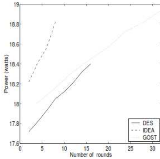
Gambar 4. Konsumsi daya vs jumlah ronde dari DES, IDEA, dan GOST Sumber: Chandramouli, dkk. (2006)
