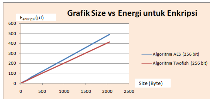
Gambar 16 Grafik konsumsi energi vs algoritma enkripsi
