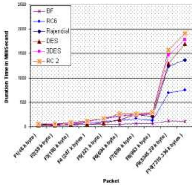
Gambar 3. Waktu enkripsi beberapa algoritma Sumber: Minaam, dkk. (2010)
