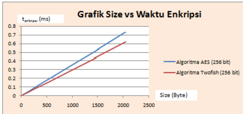
Gambar 12 Grafik size vs waktu enkripsi
