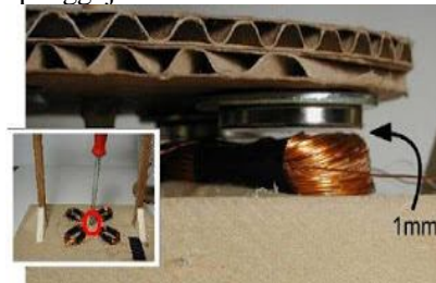
Gambar. Jarak magnet dengan lilitan
