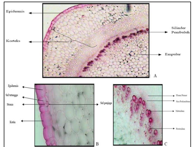
Gambar 1. Foto mikrograf irisan melintang batang anyelir : (A) struktur primer perbesaran 40x ; (B) daerah epidermis perbesaran 400x ; (C) jaringan pembuluh primer perbesaran 100x.
