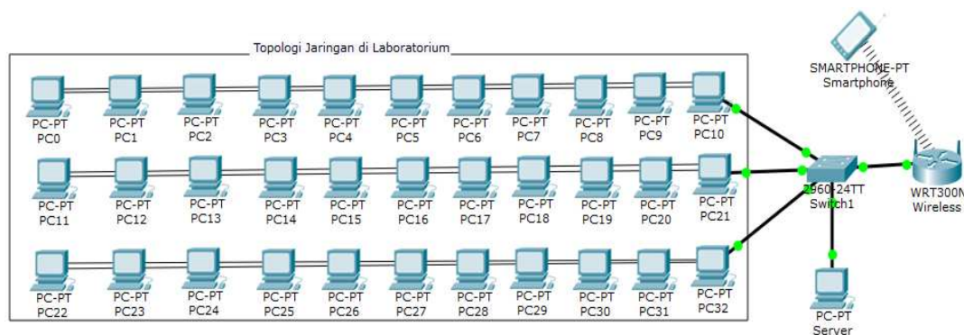
Gambar 8 Topologi Jaringan di Laboratorium (sumber: Data Olahan)
