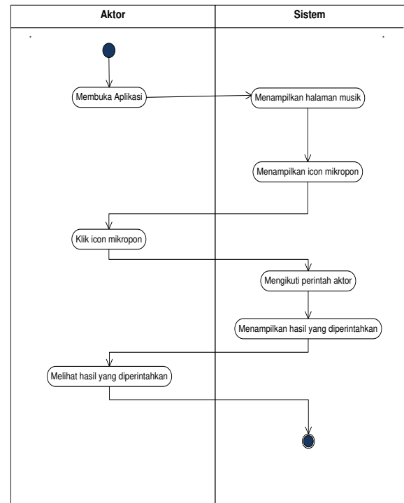
Gambar 4. Activity diagram melihat konten
