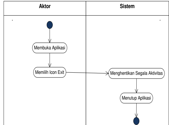
Gambar 7. Activity diagram keluar dari aplikasi
