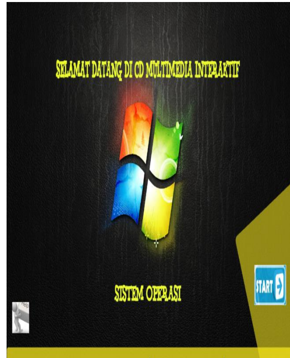
Gambar 4 . Tampilan menu
