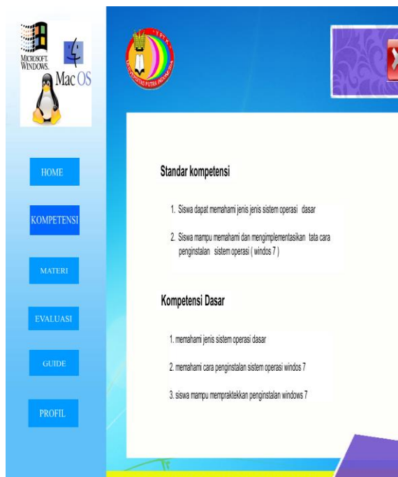
Gambar 3 . Tampilan Pendahuluan
