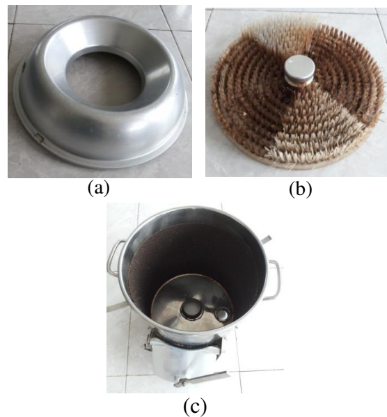
Gambar 2. Komponen utama mesin pencuci dan pengupas kentang (a) bagian penutup, (b) sikat nilan, (c) dinding silinder abrasive
