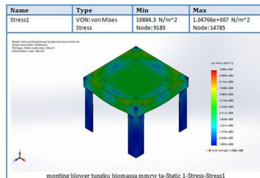
Gambar 6. Simulasi Tegangan Aktual Dudukan Fan
