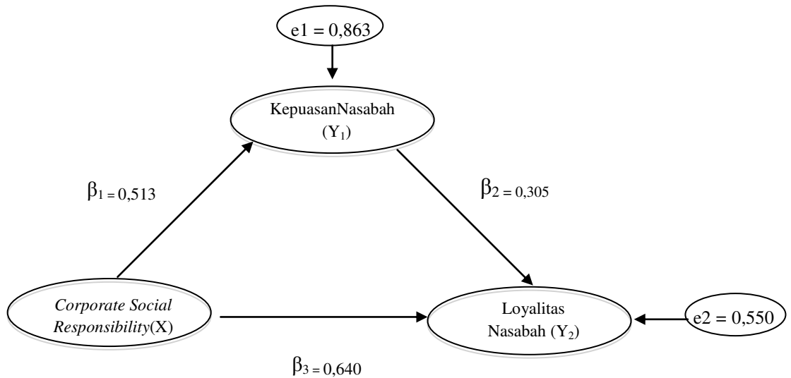
Gambar 2. Validasi Model Diagram Jalur Akhir
