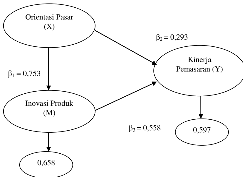
Gambar 2. Validasi Model Diagram Jalur Akhir
