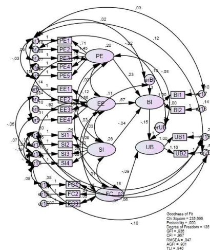
Gambar 2. Kriteria Goodness of Fit Tabel 9. Evaluasi Kriteria Goodness of Fit Indices Modifikasi
