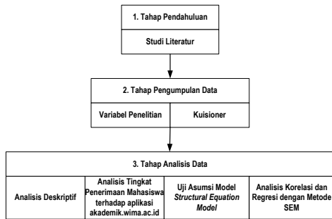
Gambar 1 Tahapan dalam Metode Penelitian
