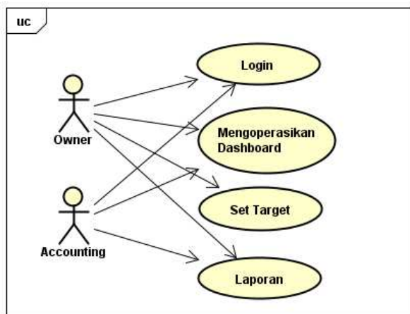
Gambar 3. Use case Dashboard Penjualan voucher pulsa elektrik
