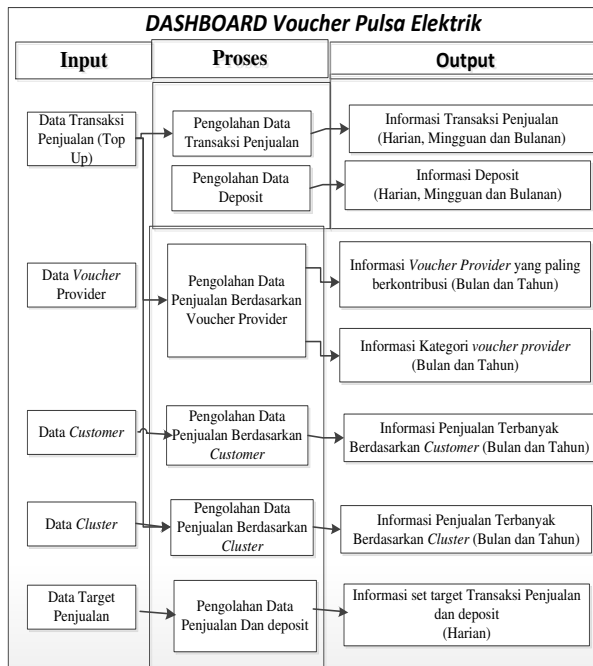
Gambar 2. IPO Dashboard Penjualan voucher pulsa elektrik
