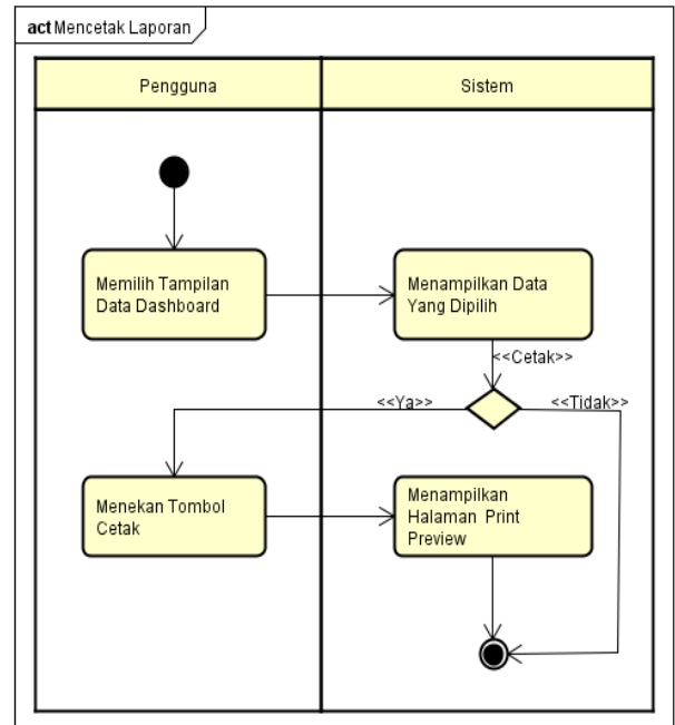
Gambar 7. Diagram Activity cetak laporan
