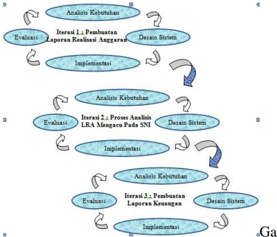
Gambar 2 Model iterasi pengembangan Agile Pada gambar 2 terapat tiga iterasi, dan didalam iterasi tersebut terdapat langkah-langkah. Penjelasan tentang iterasi di atas dijelaskan pada tabel 1 berikut ini:
