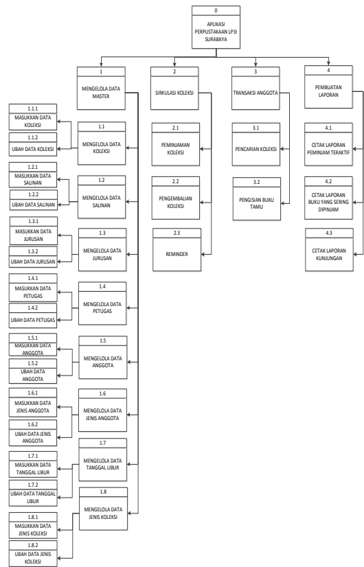
Gambar 5 Diagram HIPO
