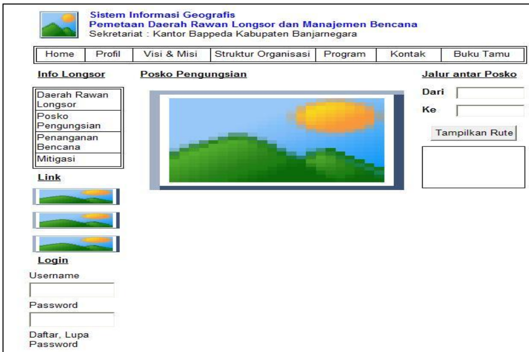
Gambar 7. Halaman Posko
