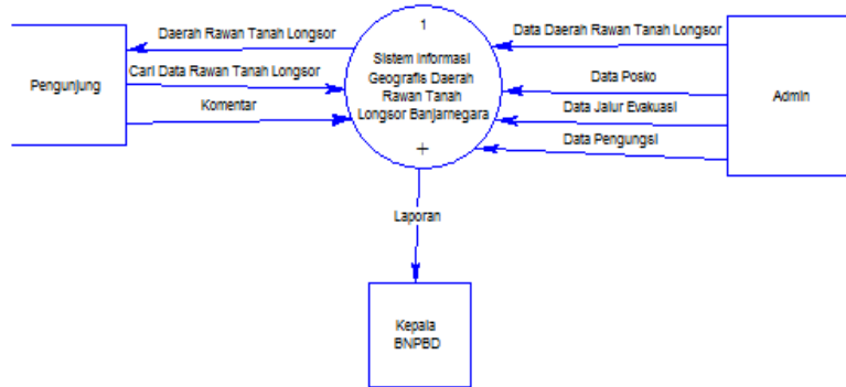
Gambar 2. Diagram konteks
