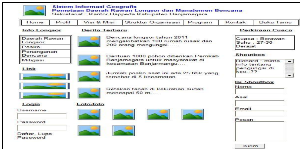
Gambar 4. Halaman Utama
