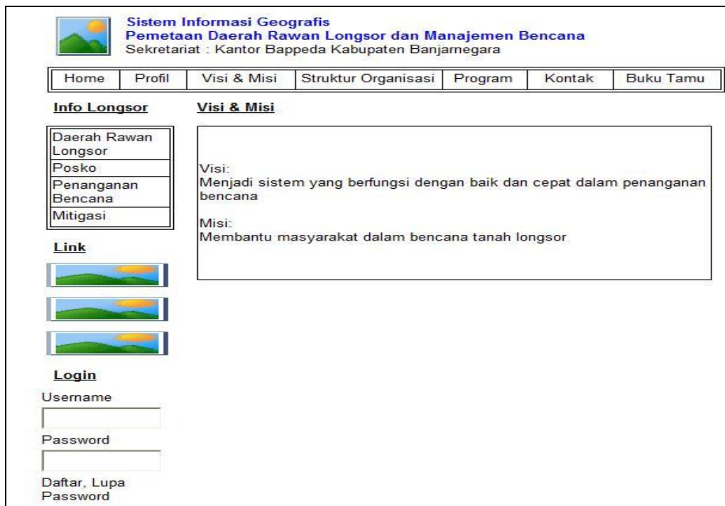
Gambar 5. Halaman Menu
