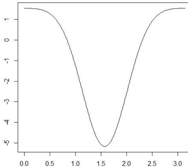
Gambar 1 Fungsi eigen dari persamaan Mathieu terkait dengan nilai eigen yang digunakan dalam artikel
