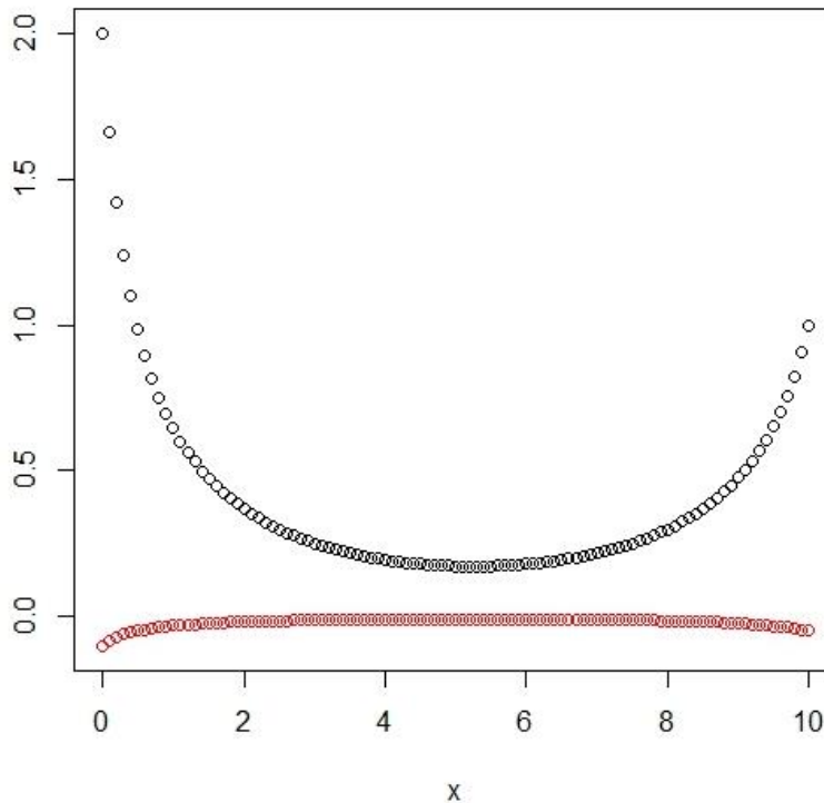
Gambar 2 Optimal y (warna hitam) dan kontrol v (warna merah) untuk Contoh 2.
