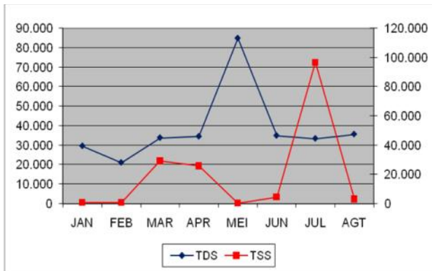
Grafik 4. Konsentrasi TDS dan TSS di Pond B tahun 2007
