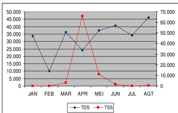
Grafik 8. Konsentrasi TDS dan TSS di Pond 4 tahun 2007
