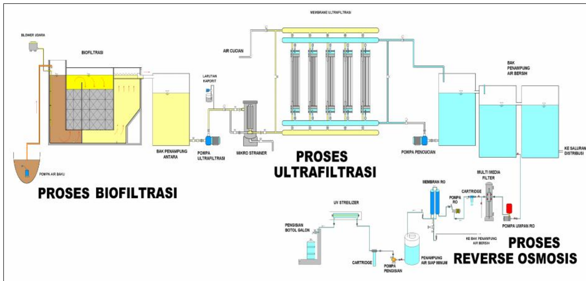
Gambar 6. Diagram pengolahan air siap minum dengan kombinasi proses biofiltrasi, ultrafiltrasi dan reverse osmosis.
