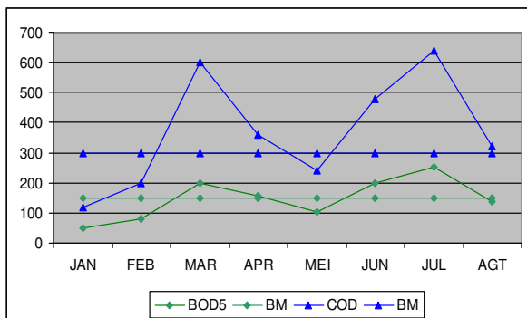
Grafik 3. Kondisi BOD dan COD Air Lumpur di Pond 4 Tahun 2007
