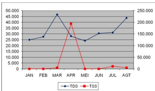
Grafik 6. Konsentrasi TDS dan TSS di Pond C tahun 2007
