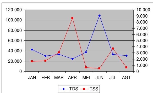
Grafik 10. Konsentrasi TDS dan TSS di Pond 5 tahun 2007
