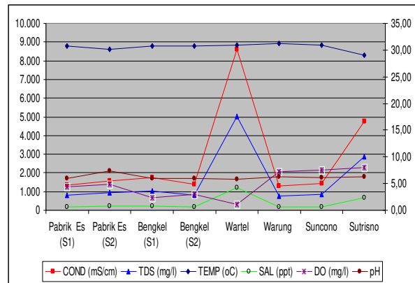
Grafik 1. Kualitas air di 7 lokasi sumur penduduk
