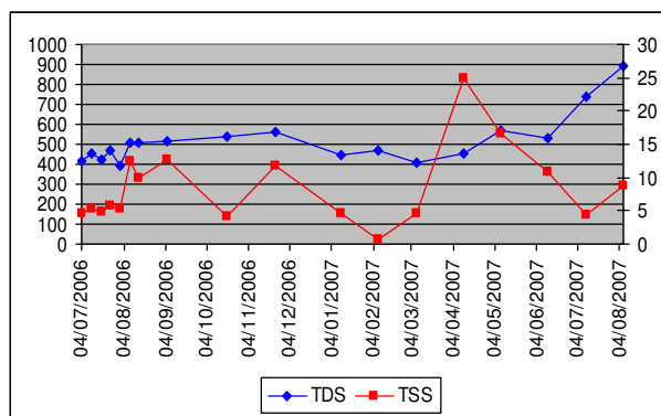
Grafik 9. Konsentrasi TDS dan TSS di Desa Mindi tahun 2006-2007
