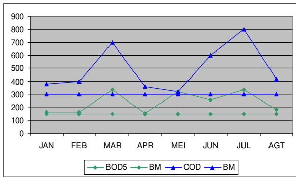
Grafik 2. Kondisi BOD dan COD Air Lumpur di Pusat Semburan Tahun 2007
