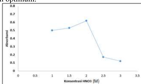
Gambar 2. Kurva optimasi asam
