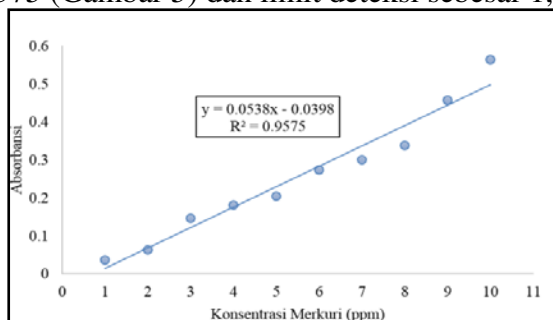
Gambar 5. Kurva hubungan antara konsentrasi merkuri terhadap absorbansi
