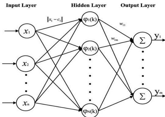
Gambar 3. Ilustrasi Proses JST RBF
