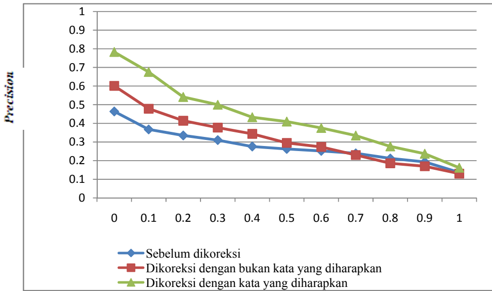
Gambar 1. Kurva rata-rata recall-precision tahap sebelum pengoreksian, tahap setelah pengoreksian dengan bukan kata diharapkan, dan tahap setelah pengoreksian dengan kata yang diharapkan.
