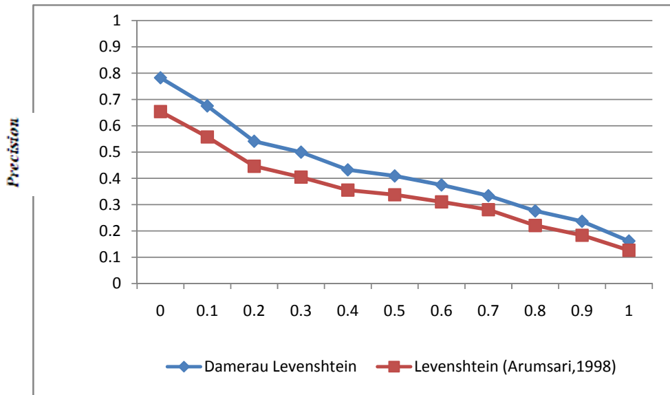
Gambar 2. Kurva recall-precision perbandingan algoritme Damerau Levenshtein dengan Levenshtein.
