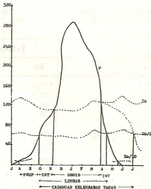
Gambar 2. Kurva keseimbangan air daerah Gerokgak berdasarkan metode Cocheme dan Franquin
