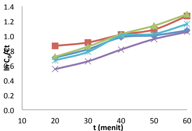
Gambar 1. Grafik hubungan \ln C_0/C_t terhadap t pada degradasi methyl orange 10 mg/L pH 4 pada berbagai konsentrasi SO_4^{2-}
