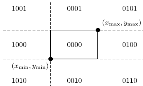
Gambar 6 Kode 4 bit algoritma Cohen-Sutherland (klawonn, 2012)
