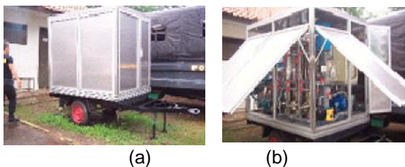
Gambar 18. Contoh Unit Pengolah Air Jenis Mobile, ditarik untuk mengolah air keruh kapasitas 10 s.d. 20 m 3 /hari.
