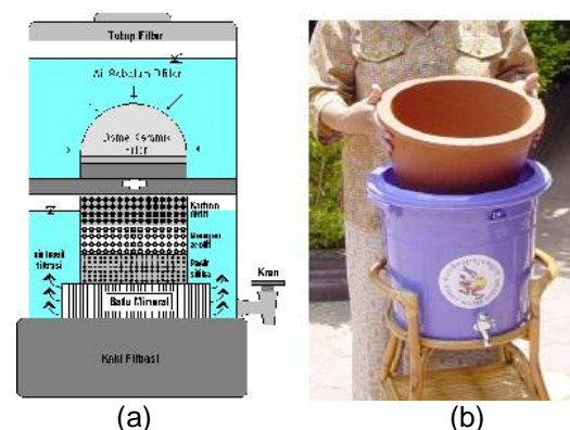
Gambar 3. Saringan Keramik. (a) Tipe Dome dan (b) Tipe Mangkuk.
