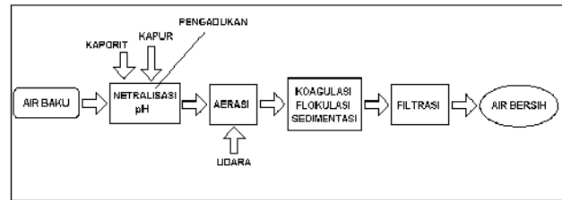
Gambar 6. Diagram Proses Pengolahan Air Sederhana TP2AS.
