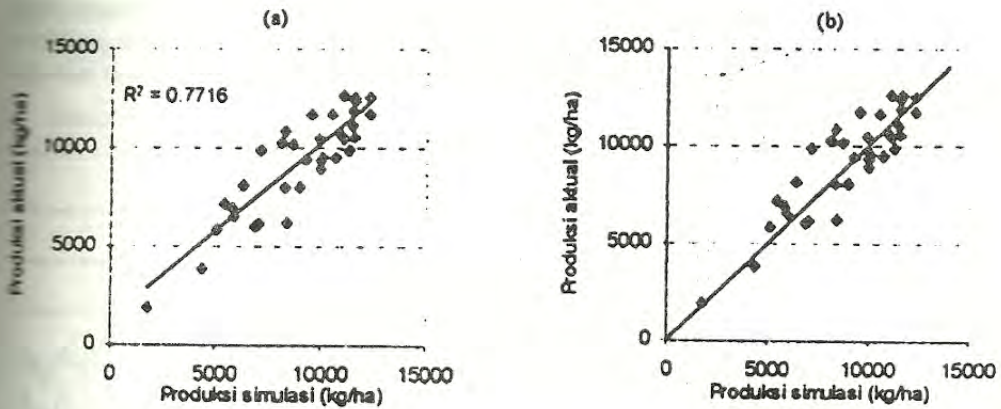
Gambar 5. Diagram pencar hubungan produksi aktual dengan simulasi (a) dan terhadap garis 1:1 (b) pada pengujian model.
