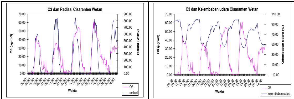
Gambar 5. Fluktuasi radiasi dan kelembaban udara dengan konsentrasi O 3
