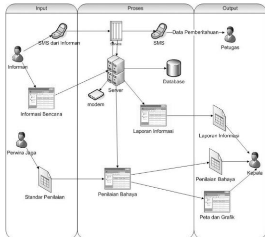
Gambar 2 Arsitektur Aplikasi
