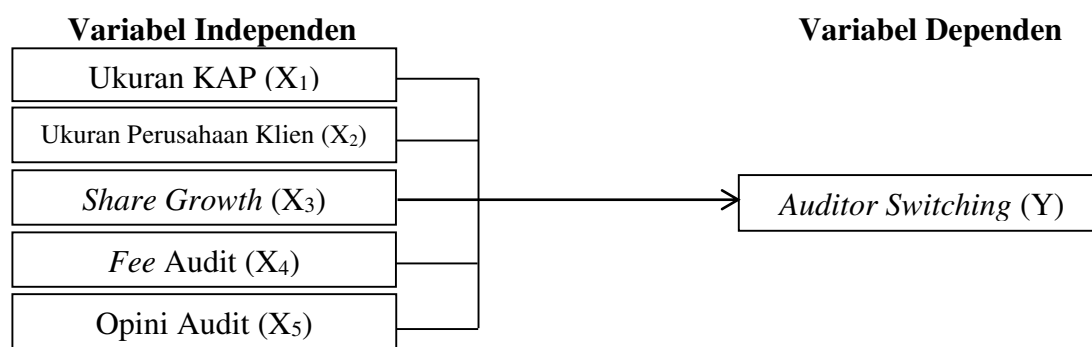
Gambar 1. Kerangka Konsep
