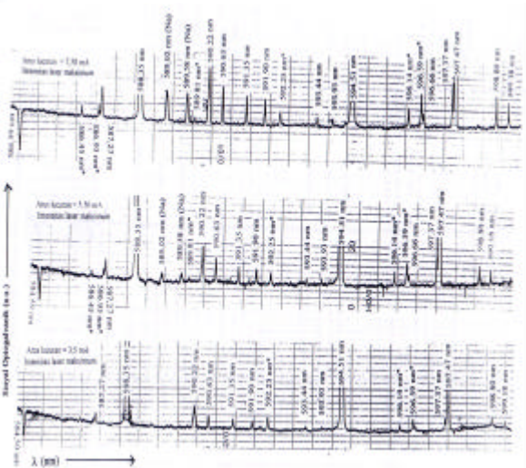
Gambar 4. Spektrum optogalvanik atom Ne pada intensitas laser pengeksitasi yang tetap (100%) dengan arus lucutan yang divariasikan ( I_{\text{lucutan}} = 3,5; 5,5; 7,5 \text{ mA} ).
