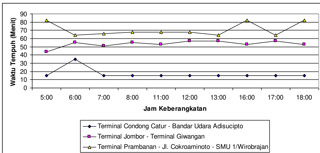
Gambar 13. Pengujian Waktu Tempuh Pencarian Rute Tercepat
