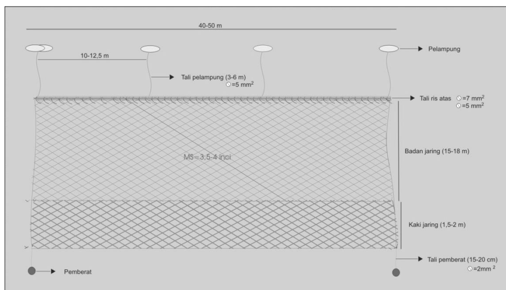
Gambar 2 Konstruksi jaring insang.
