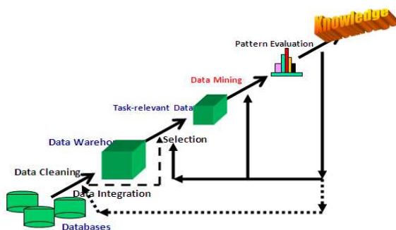
Gambar 1. Proses penemuan pengetahuan dalam database / KDD (Han & Kamber, 2006)
