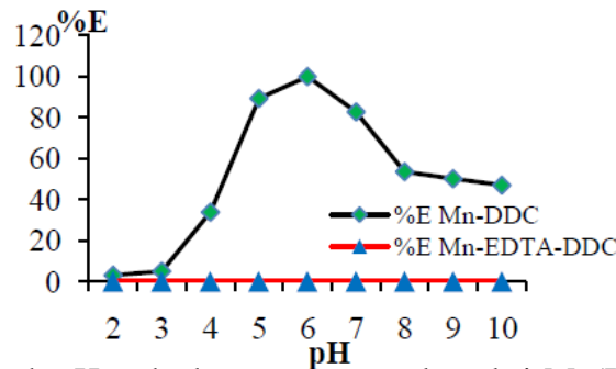
Gambar 8. Pengaruh pH terhadap persentase ekstraksi Mn(DDC) 2 dan penopengan dengan EDTA
