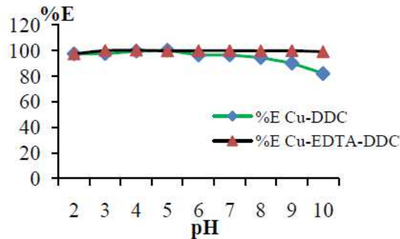
Gambar 7. Pengaruh pH terhadap persentase ekstraksi Cu(DDC) 2 dan penopengan dengan EDTA
