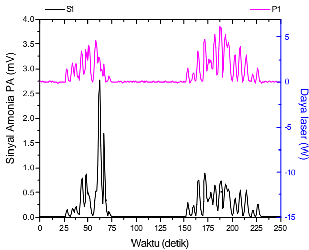
Gambar 4. Grafik scanning seluruh garis laser CO 2 pada daerah 10P dan 10R untuk gas amoniak murni dengan konsentrasi 7 ppm
