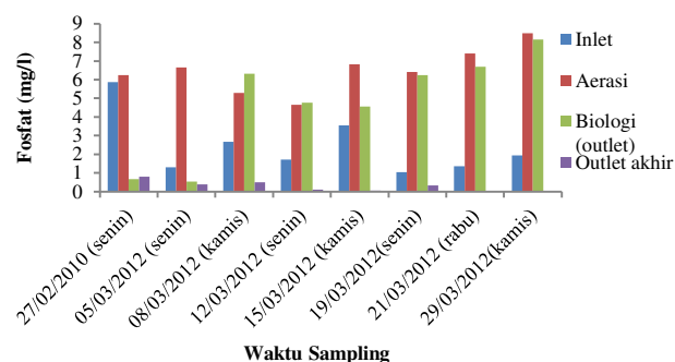
Gambar 8. Perubahan kandungan nilai fosfat air limbah bulan Maret 2012
