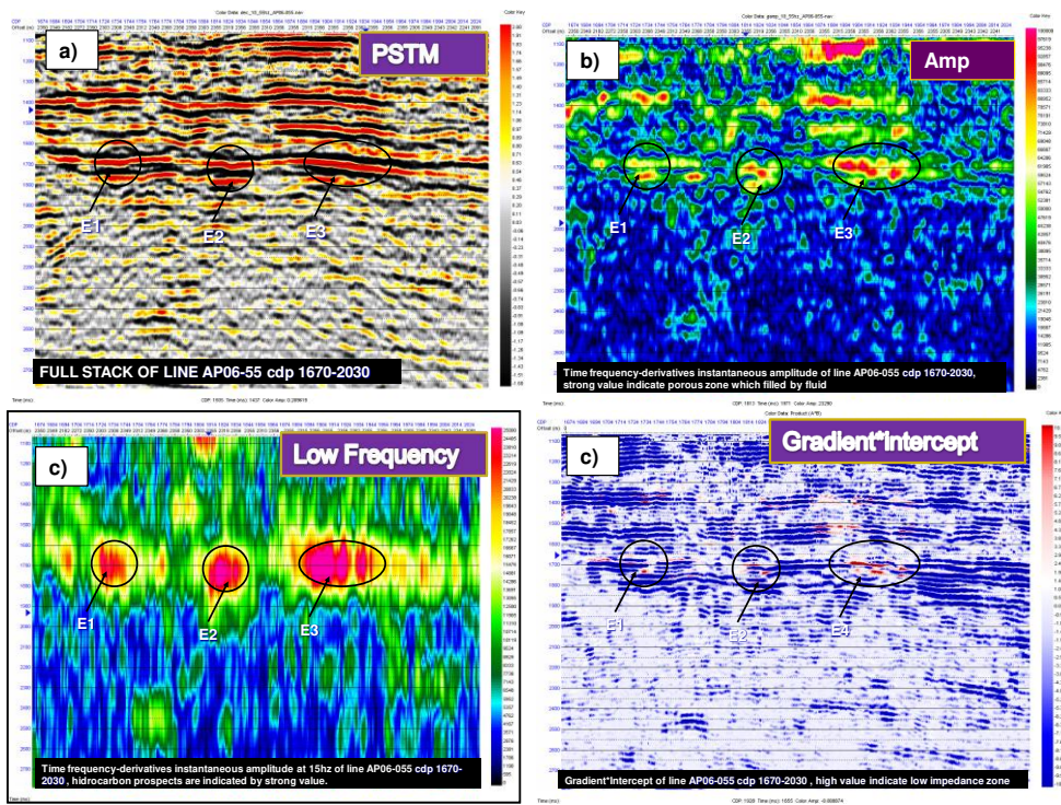
Gambar 6. a) Penampang Seismik PSTM, b) atribut amplitudo sesaat, c) atribut amplitudo gradient waktu-frekuensi 15hz d) atribut gradient*intercept pada lintasan prospek
