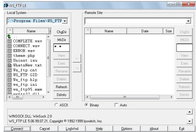
Gambar 2. Tampilan WS-FTP
