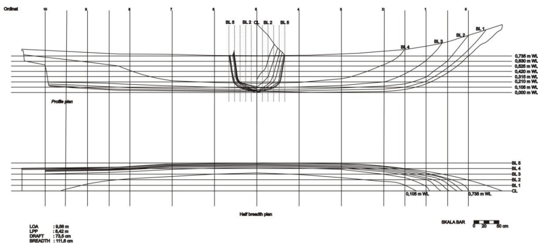
Gambar 11 Rencana garis perahu Kahuripan Nusanantara
