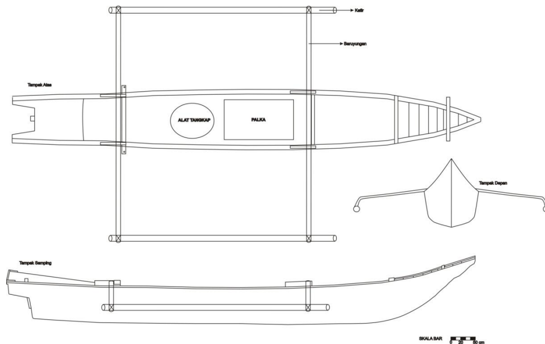
Gambar 10 Rancangan umum perahu Kahuripan Nusantara
